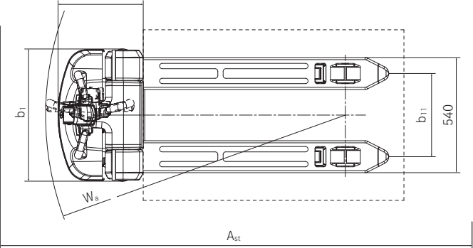
ECH 15 vista superior
