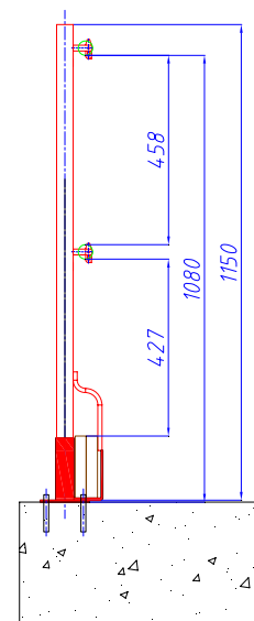
Dimensiones de montaje formado por Soporte + E-1150-14
